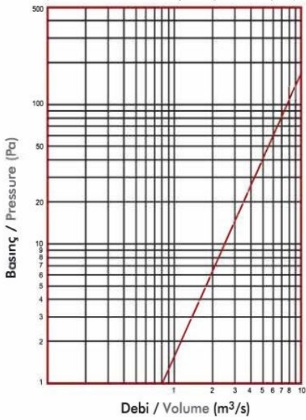
Basınç Kaybı / Debi Grafiği Pressure Drop / Volume Graph
